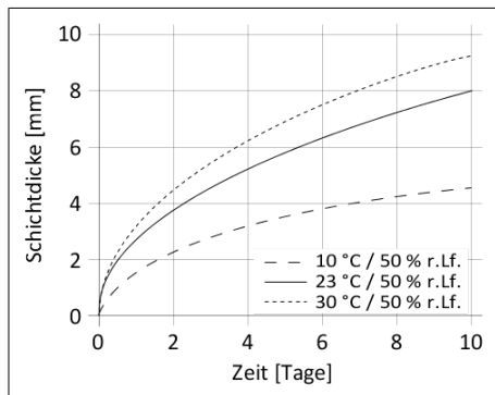
Diagramm 1: Durchhärtengeschwindigkeit Sikaflex®-591
